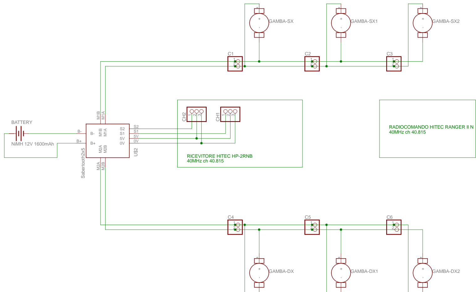
SCHEMA CABLAGGIO cespuglio Aggiornato al : 6 jun 2008
